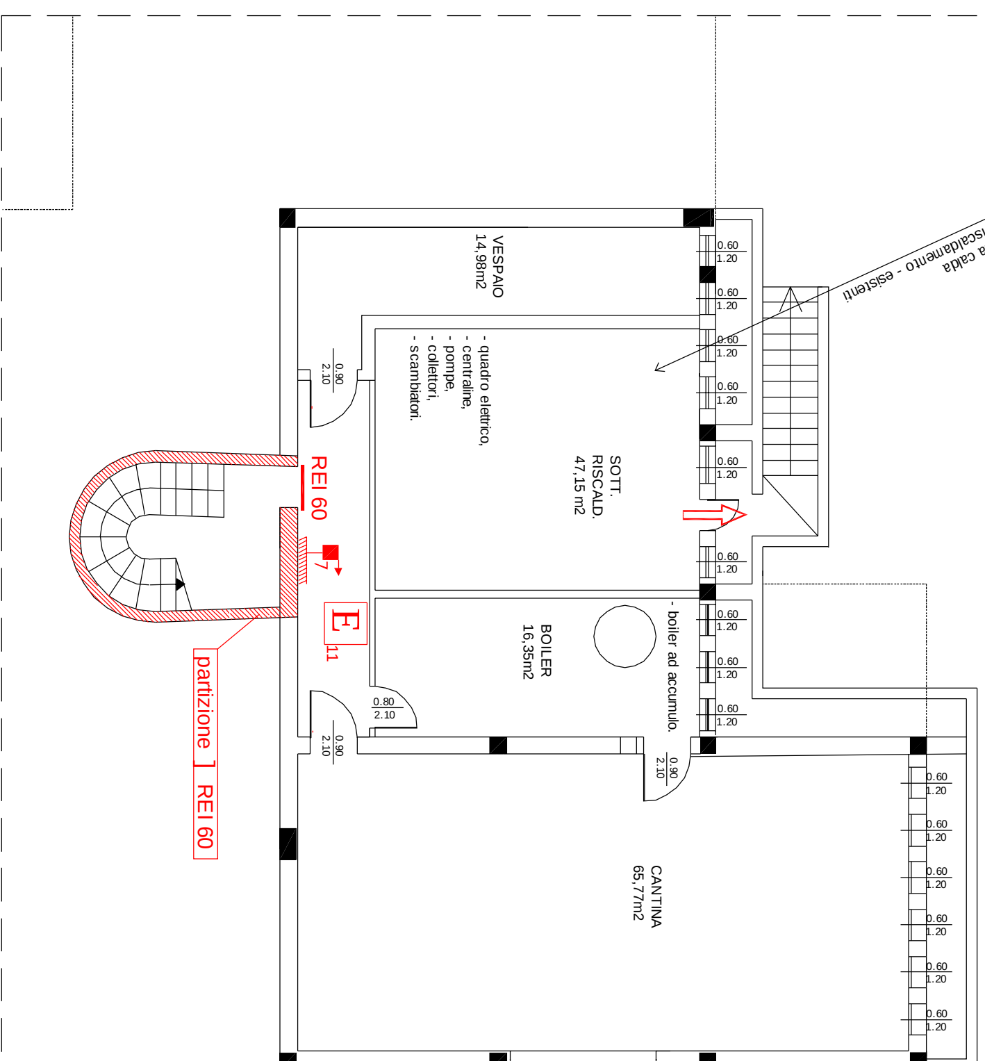
Scuola Materna - Piano Interrato ATTIVITA' 67.2.B
