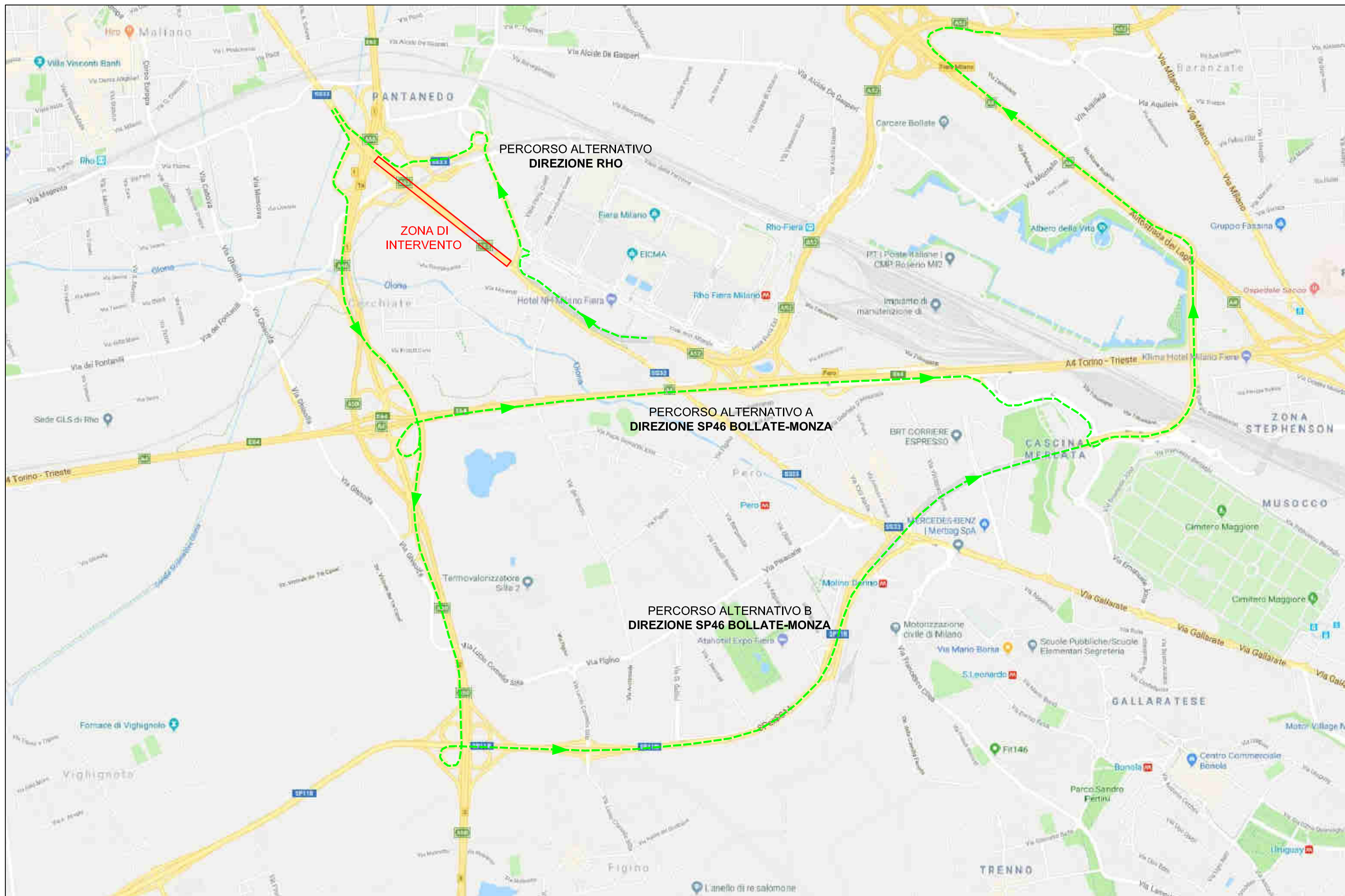
A50 Tangenziale ovest - Intervento di ripristino dell'impermeabilizzazione della galleria Cerchiarello Planimetria dei percorsi alternativi
